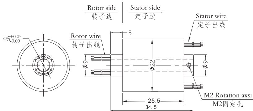
12路不带法兰规格图纸
