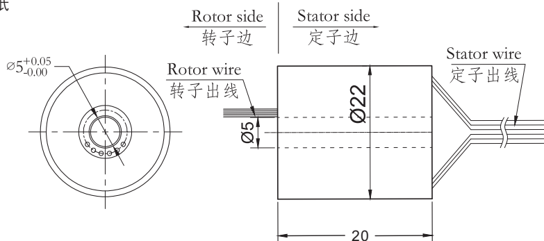
12路带法兰规格图纸
